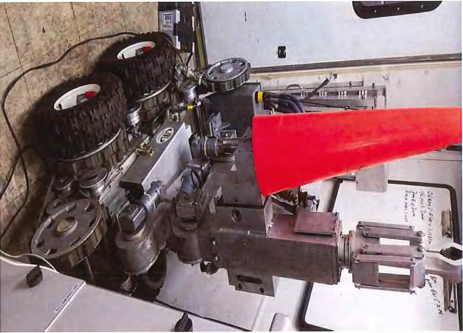
EOD5- Robot Gripper
